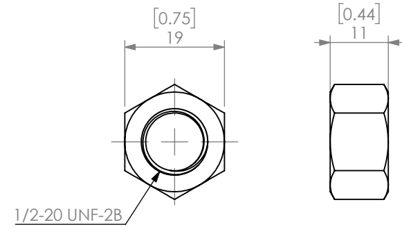
570-ADJ nut
