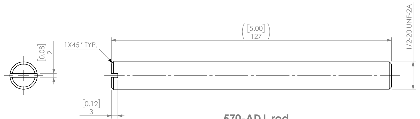
570-ADJ rod
