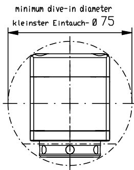
Ansicht Y
