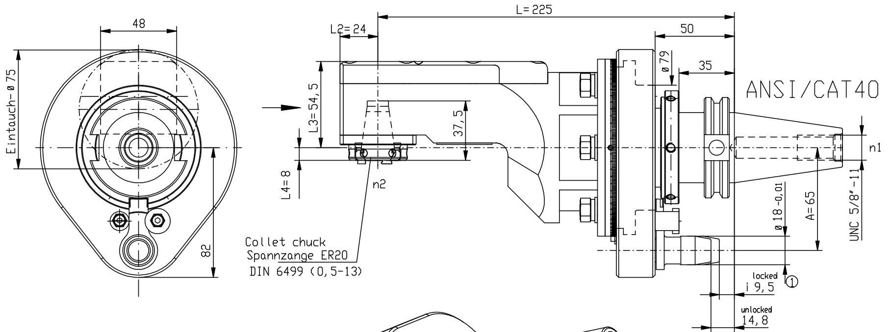
Ansicht Y
