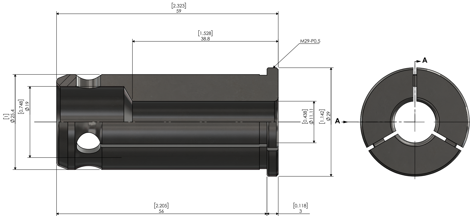
SECTION A-A
