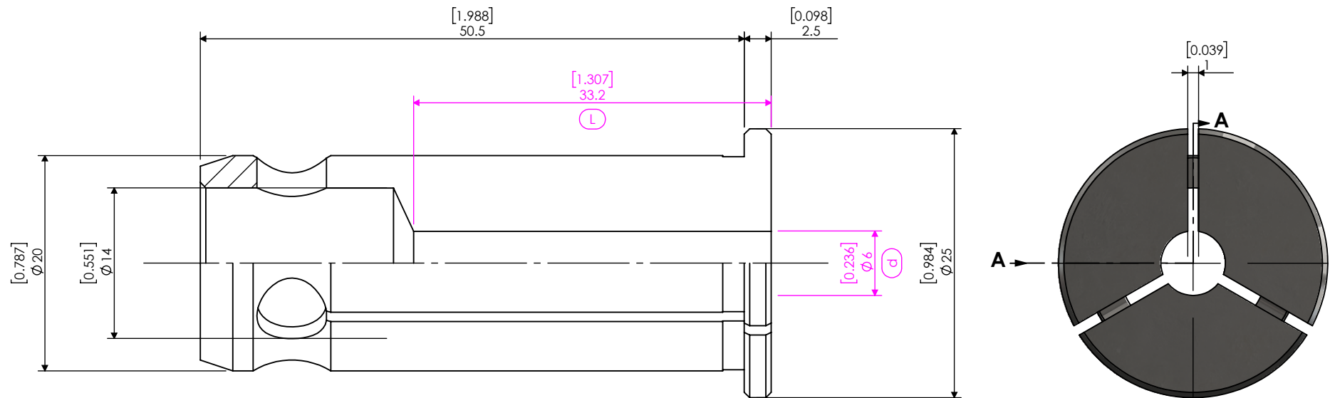
SECTION A-A
