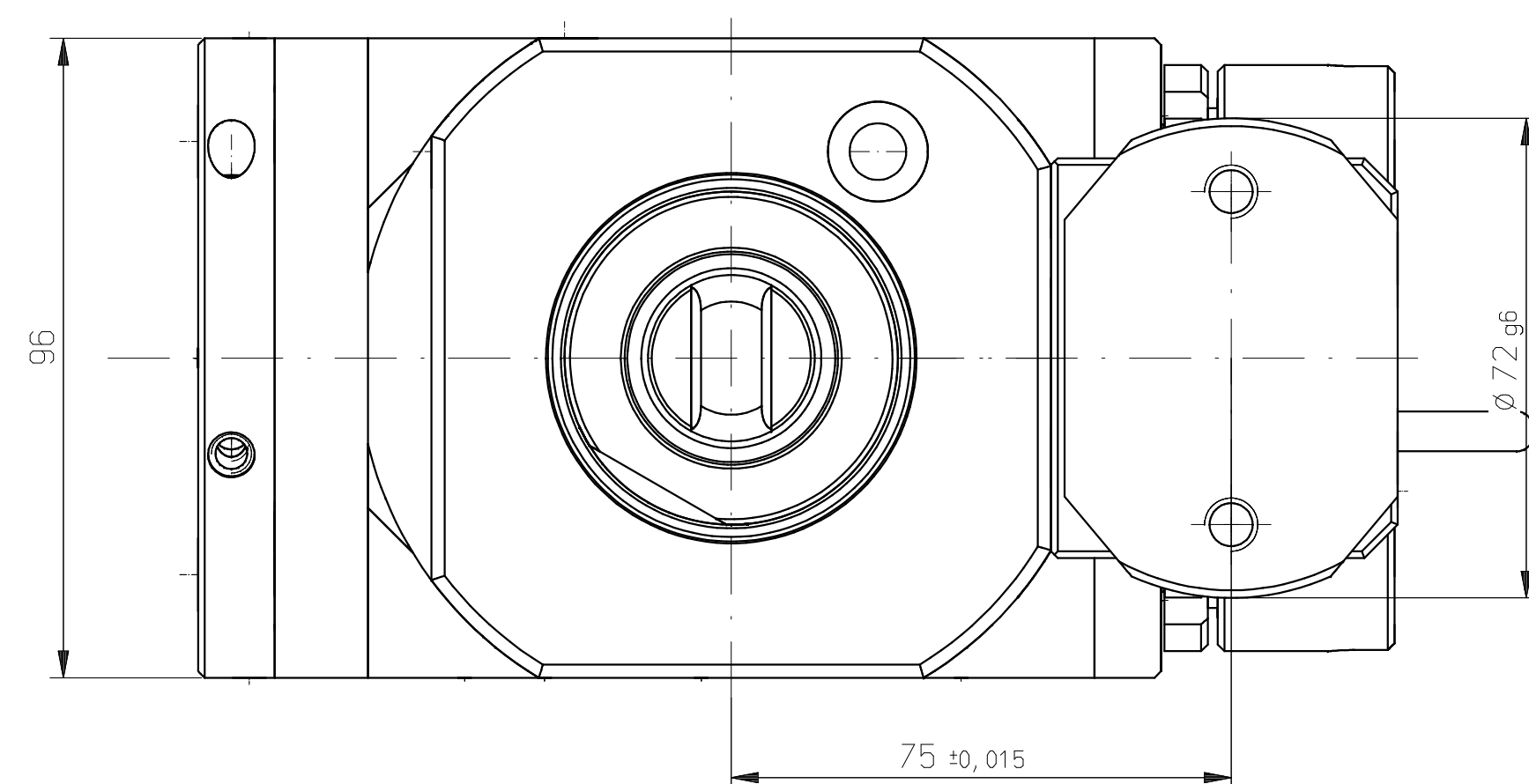
Ansicht X
