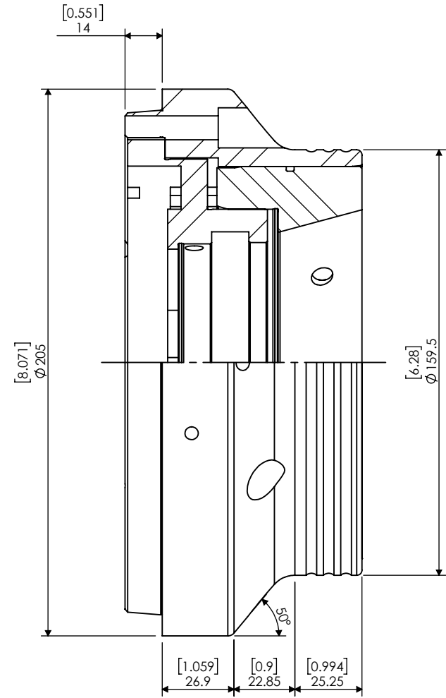
SECTION A-A
